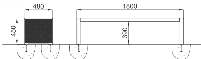
4 scellements \varnothing 12x150
